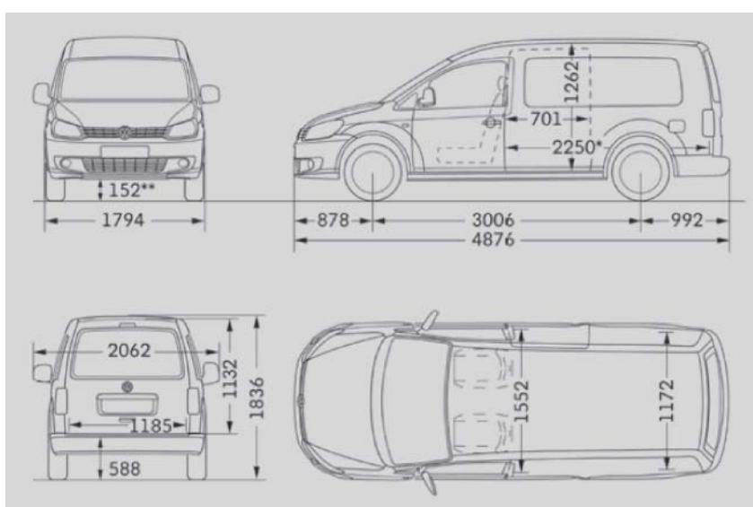
Caddy Maxi Van long wheelbase
